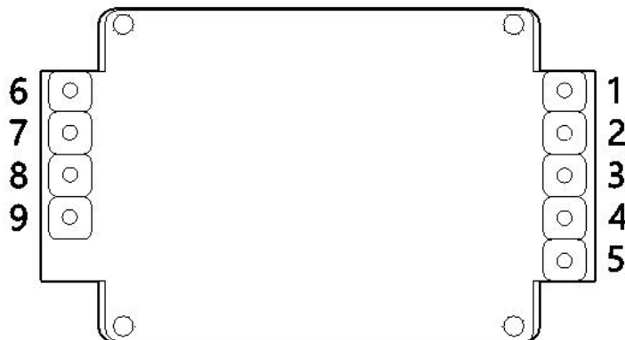
图1 引脚定义图
