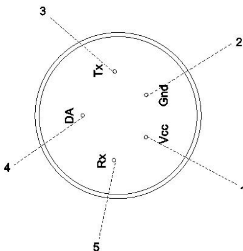
图1 引脚定义图
